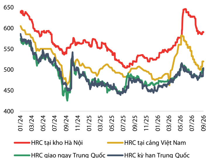
Hình 13: Diễn biến giá HRC tại Trung Quốc và Việt Nam (USD/tấn)
